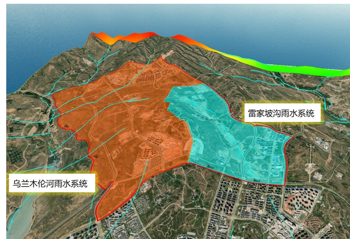
图 6.3 康巴什北区雨水分区
