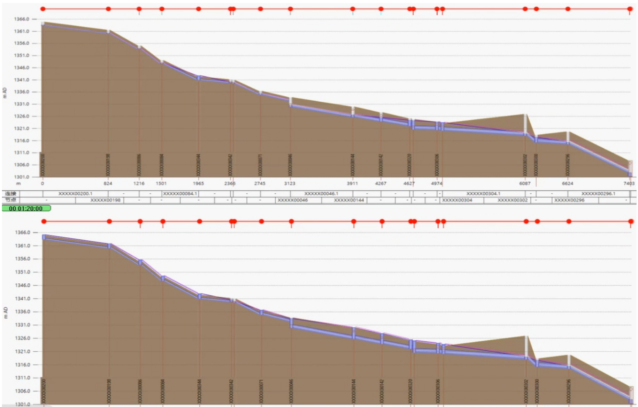
图 4.4 特征管道 0.5a 一遇和 2a 一遇降雨下水管道纵断示意图
