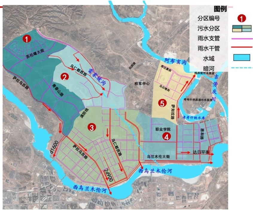
图 3.3 康巴什排水流向图
