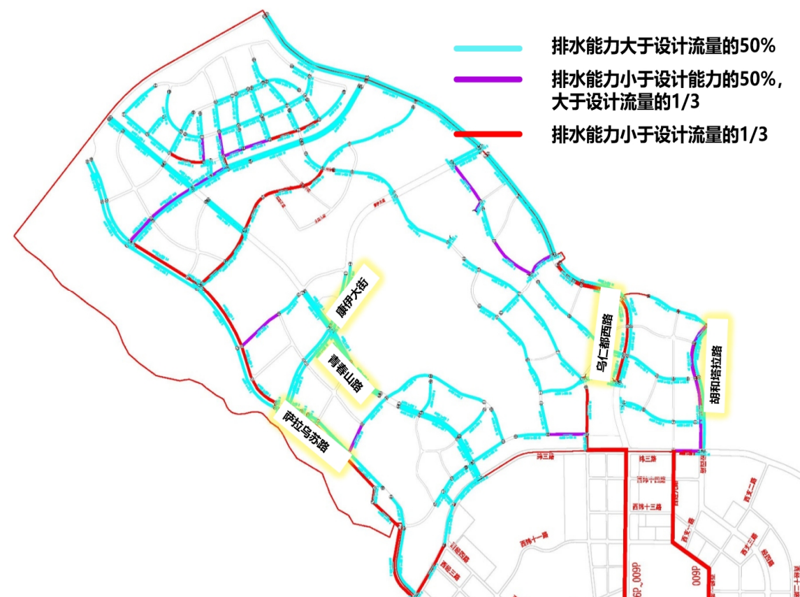
图 4.3 康巴什北区现状雨水管道排水能力校核
